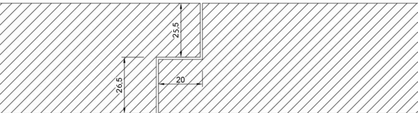
Połączenie ościeżnicy drzwi z obróbką
